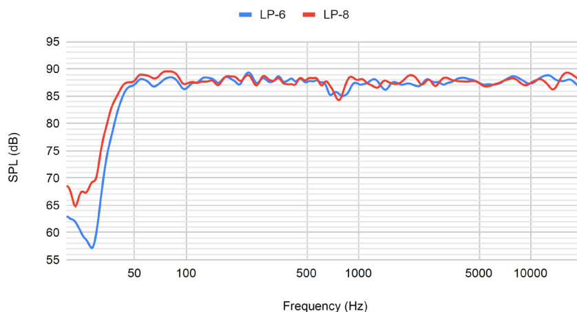
Частотная характеристика LP—6 и LP—8 по оси
